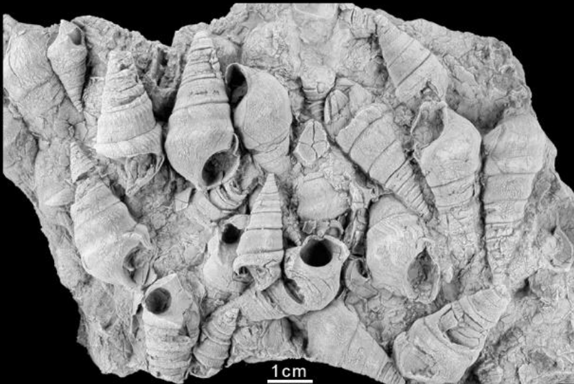
Lumaquela de Paraglauconia (gasterópodos), foto de campo (arriba) y teñida con cloruro amónico sublimado (abajo).
