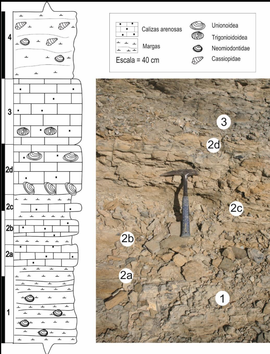
Detalle de columna estratigráfica del yacimiento de Los Cayos (Cornago, La Rioja).
